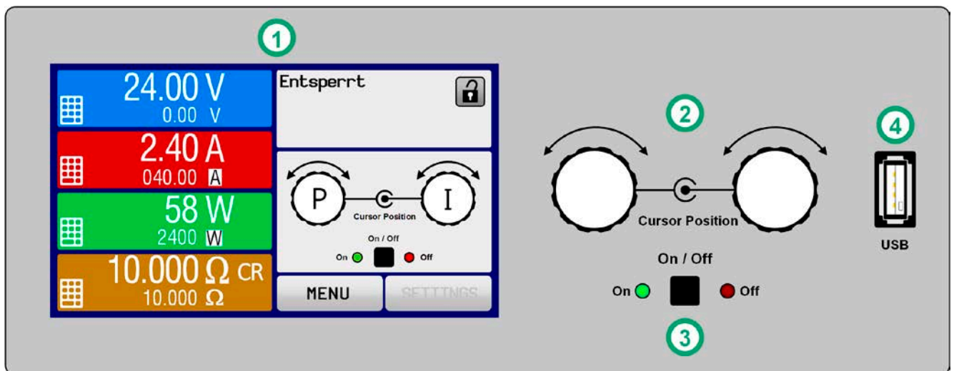
Bild 11- Bedienfeld
