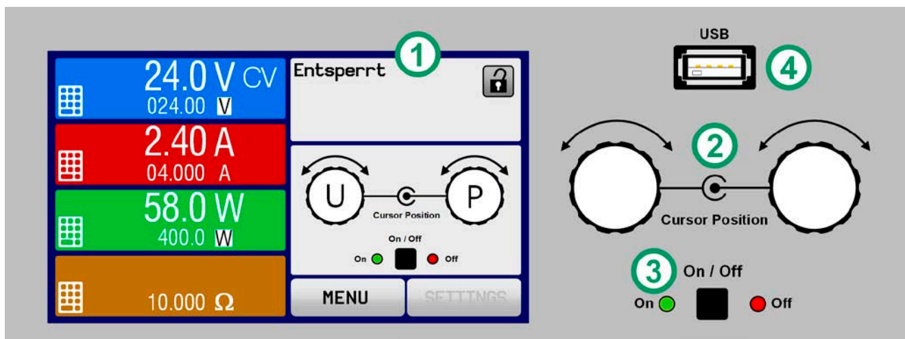
Bild 6- Bedienfeld
