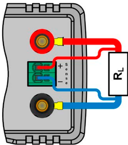
Bild 13 - Prinzipbeispiel Fernföhlungsverdrahtung
