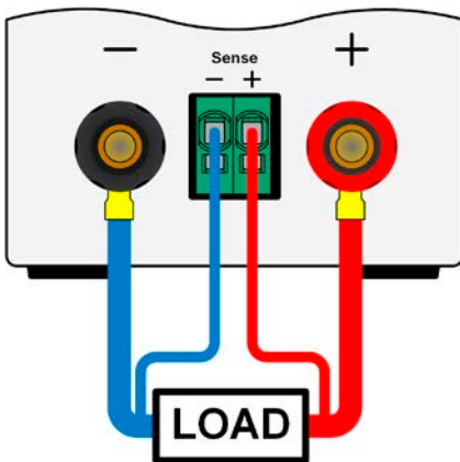
Bild 7 - Prinzipbeispiel der Fernfühlungsverdrahtung
